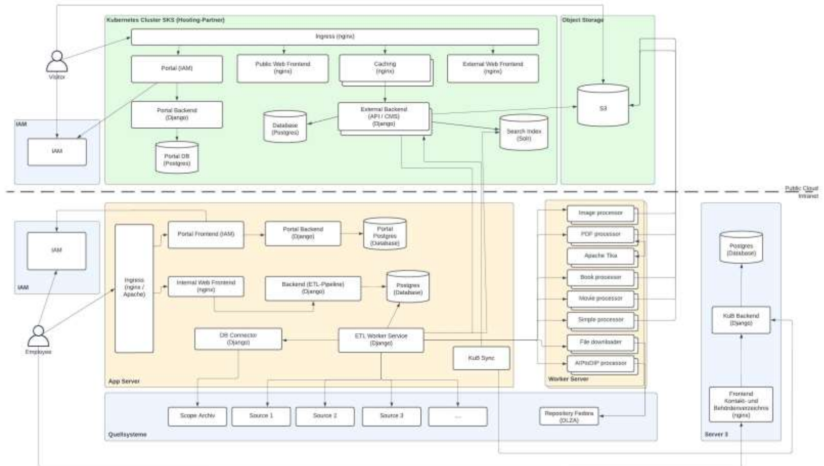
Architekturdiagramm
